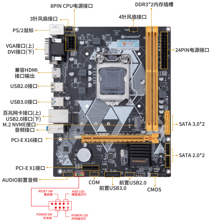
图1-1 H81主板图解
