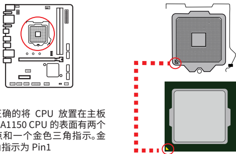
图2-6 CPU安装
